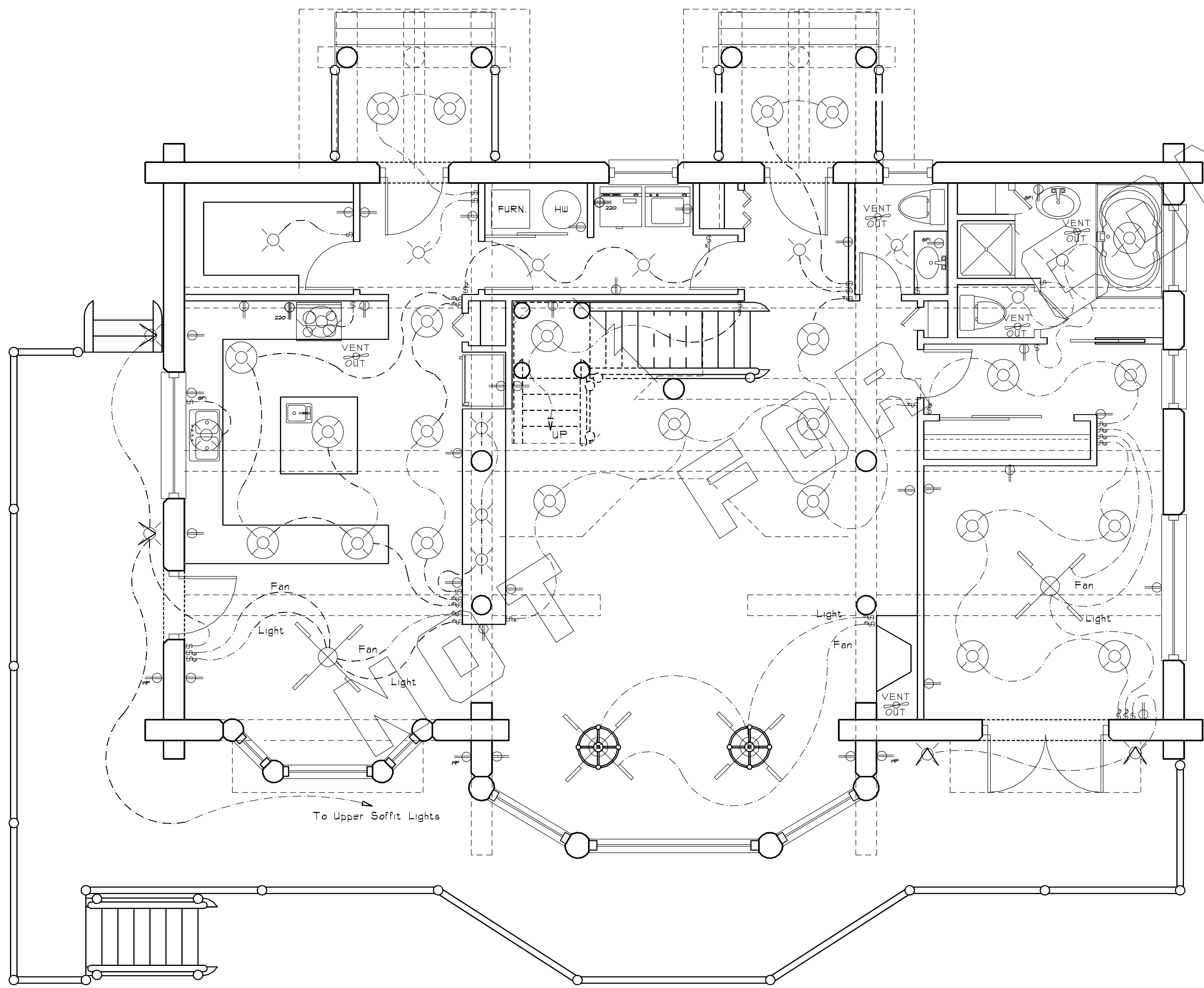
1 MAIN FLOOR ELECTRICAL A.12 N.T.S.
